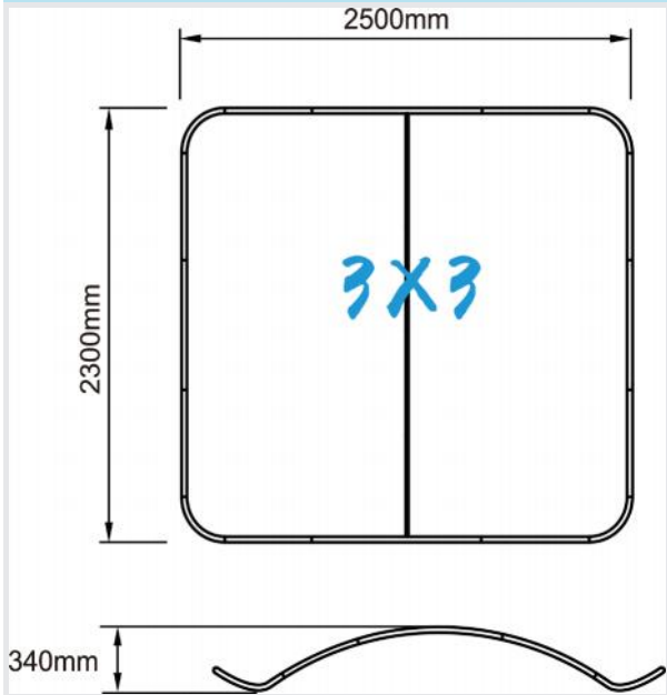
Frame 3x3
