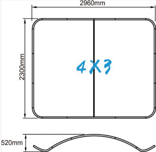
Frame 4x3
